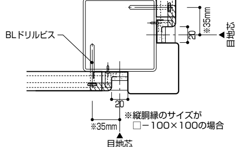
出隅部（目地幅20mmの場合）
