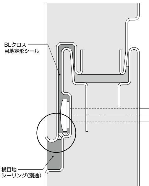
【A-A断面図】
