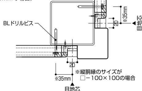
出隅部（目地幅20mmの場合）
