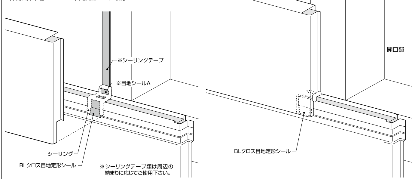
B部開口部下端のBLクロス目地定形シール取付
