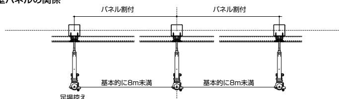
図2 足場控えと外壁パネルの関係
