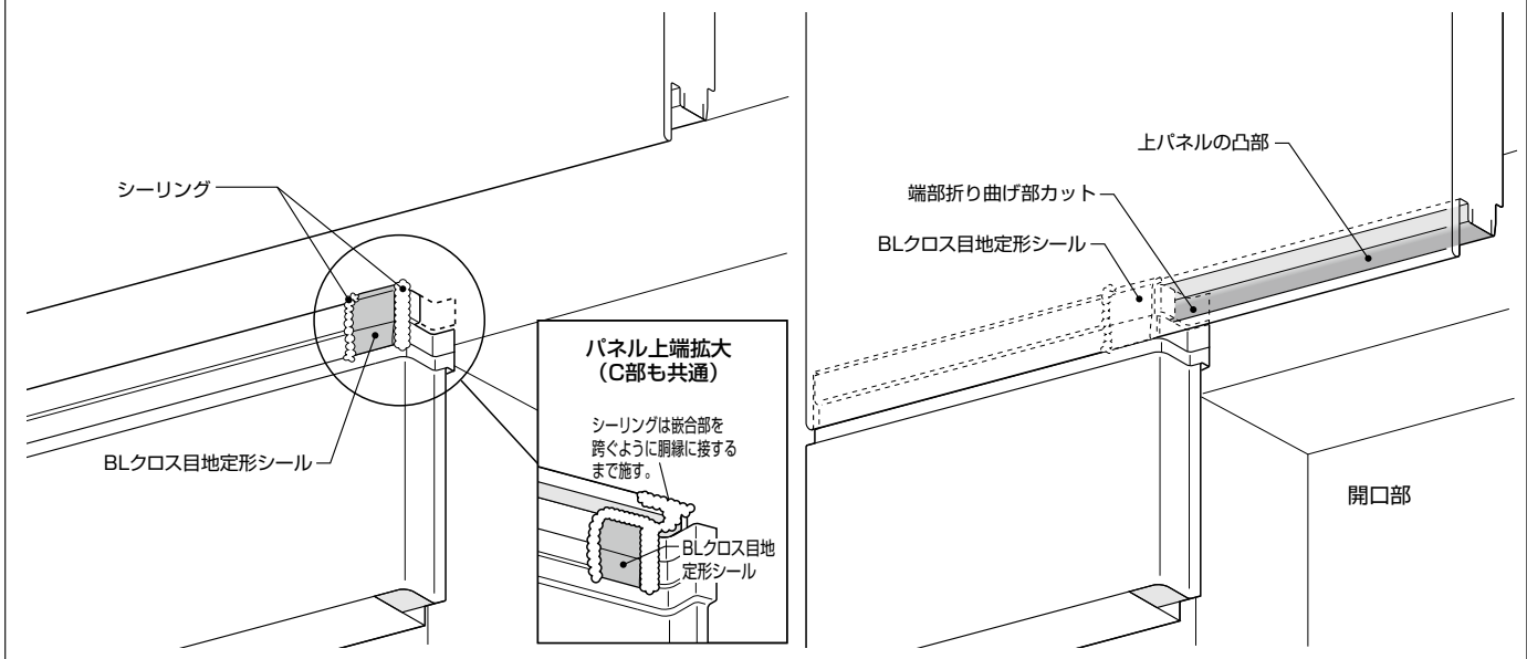
A部開口部上端のBLクロス目地定形シール取付
