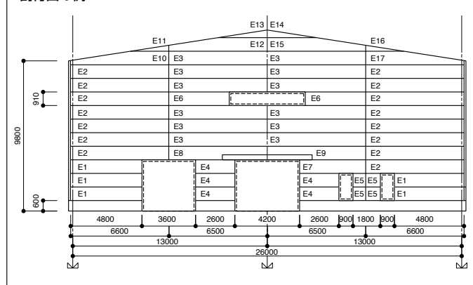
割付図の例
