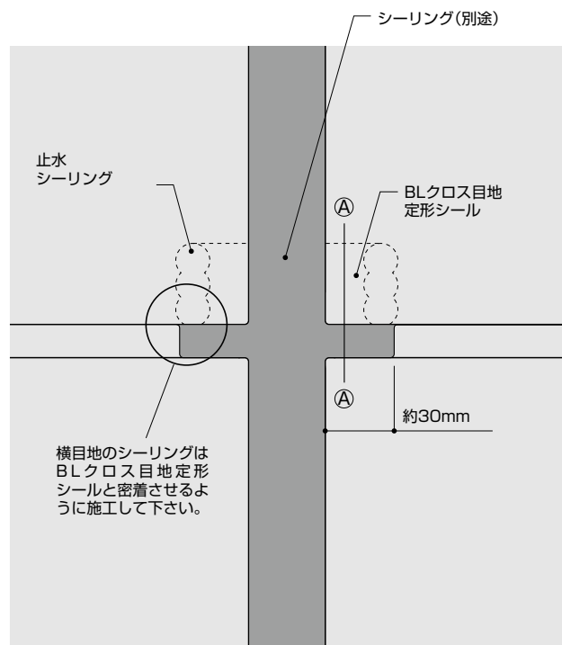
十字目地部正面図
