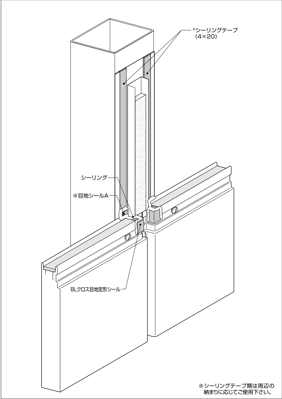
縦ジョイント溝型AとTパッキンの関係
